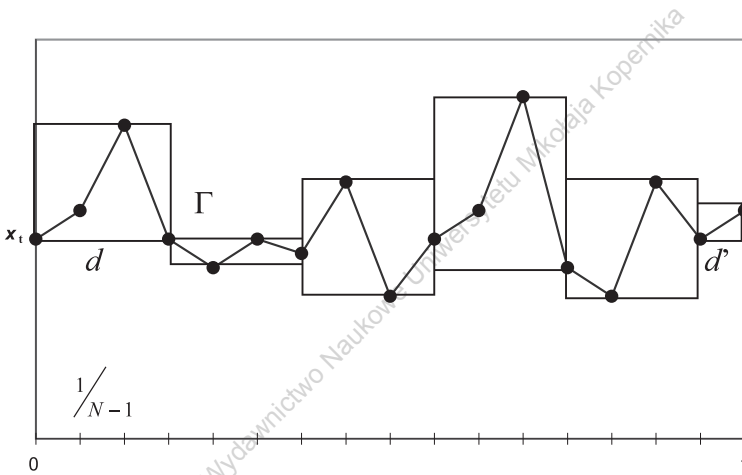
Rysunek 2. Tworzenie zbioru \Gamma w metodzie segmentowo-wariacyjnej dla m = 4
